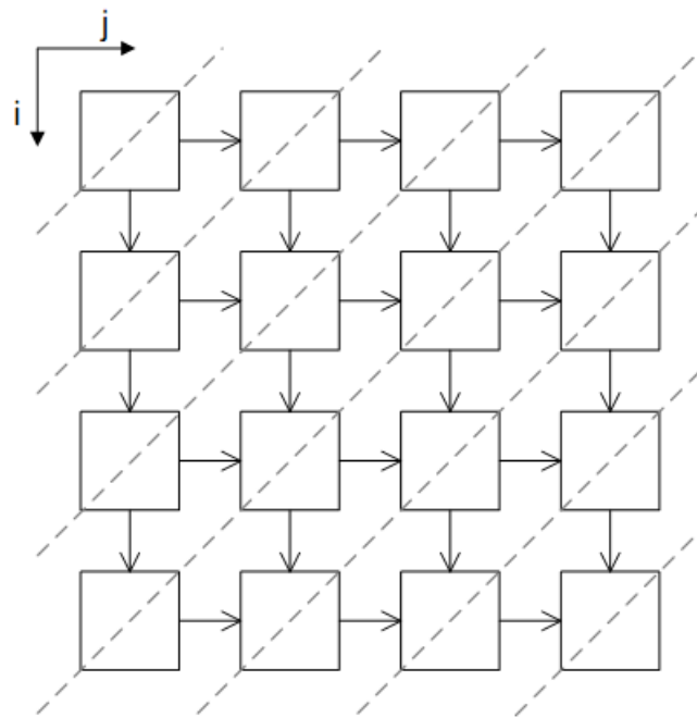
Рис. 4: Разделение итерационного пространства на гиперплоскости. Внутри одной гиперплоскости элементы могут считаться параллельно.
