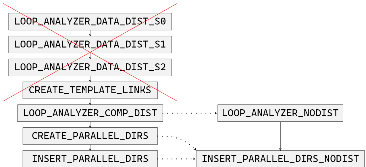
Рис. 2: сравнение схемы работы проходов режима распараллеливания с распределением данных (слева) с новым режимом распараллеливания на общую память (справа).
