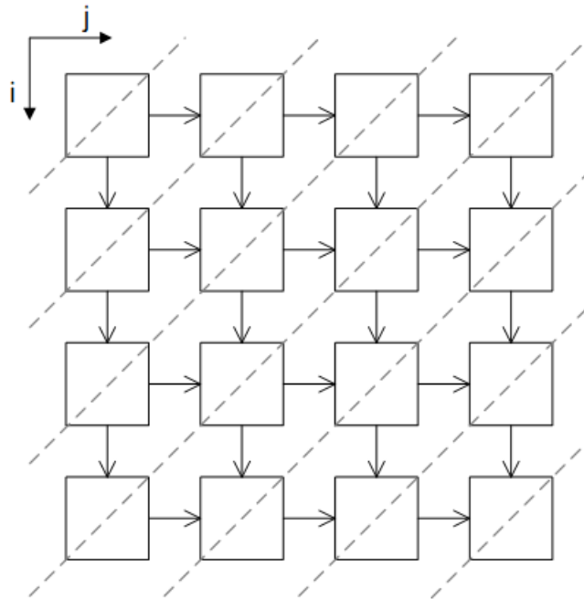
Рис. 5: разделение итерационного пространства на гиперплоскости. Внутри одной гиперплоскости элементы могут считаться параллельно.
